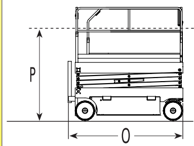
Macchina chiusa con ringhiere abbassate Stowed machine with folded-down rails
