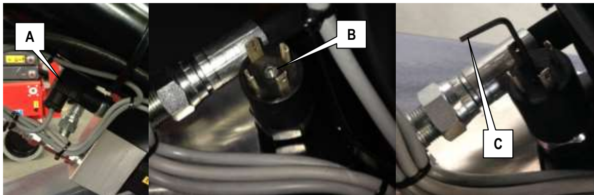
7-9: Standardtype belastningskontrol
