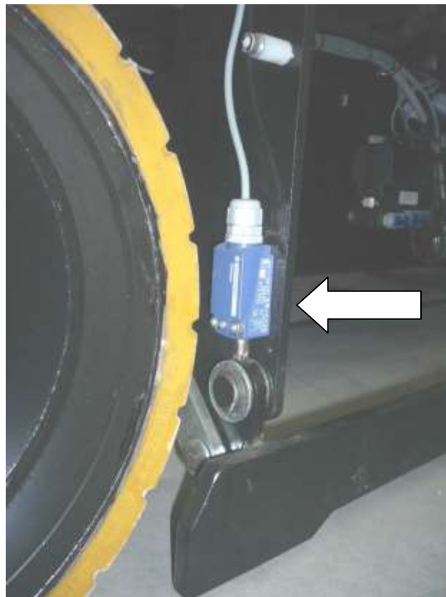
7-12: MPT1 mikroafbryder
