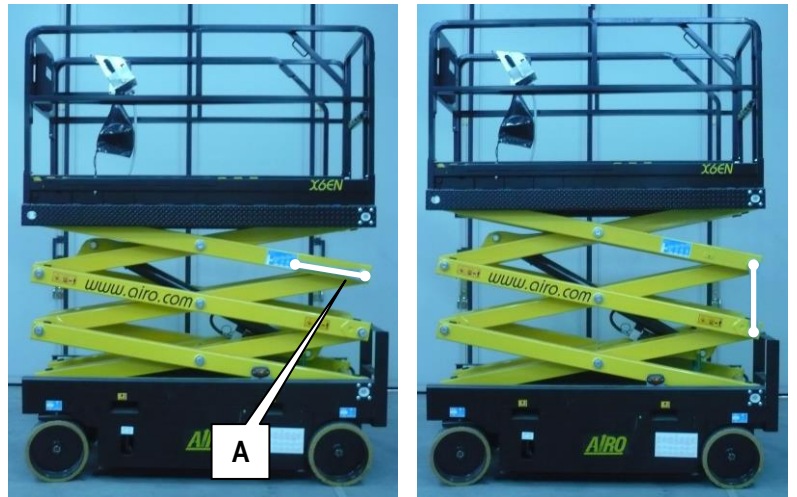
7-1: Scherensperrung X8 EN, XS7 E RESTYLING
