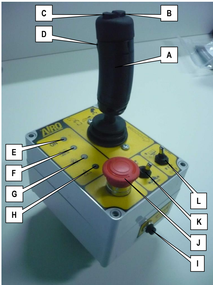
5-1: Plattformbedienpult
