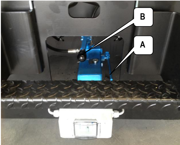
5-8: Manuelle Absenkung vom Boden
