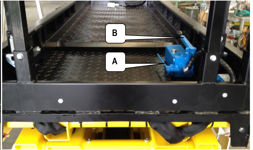
5-9: Manuelle Absenkung von der Plattform
