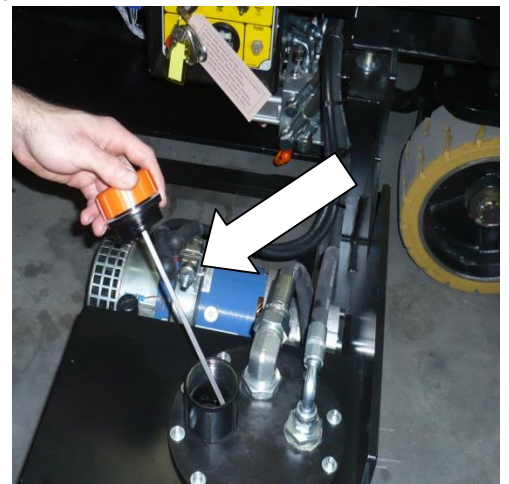
Bouchon de contrôle du niveau de l'huile de la série XSE RESTYLING
