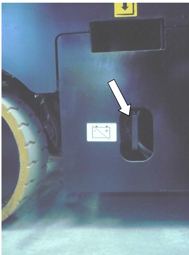
5-5: Connecteur de puissance série "X"
