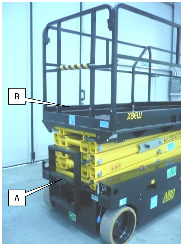
5-4: Position d'accès/abandon à la plate-forme
