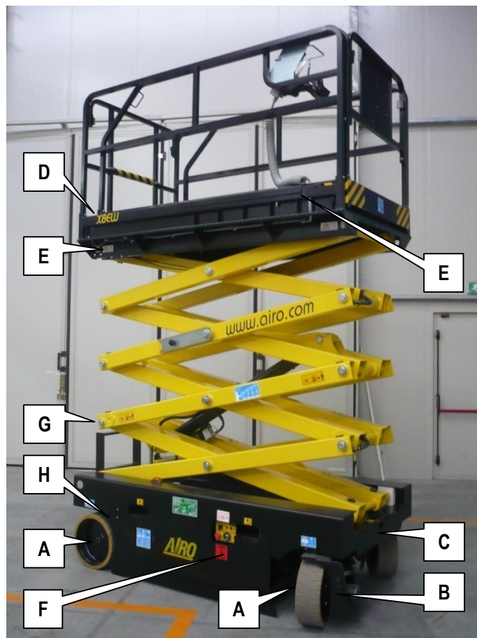
7-4: Emplacement des composants à régler
