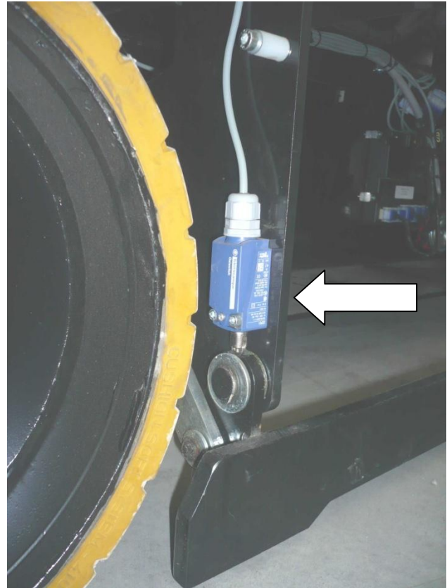
7-11: Minirupteur MPT1
