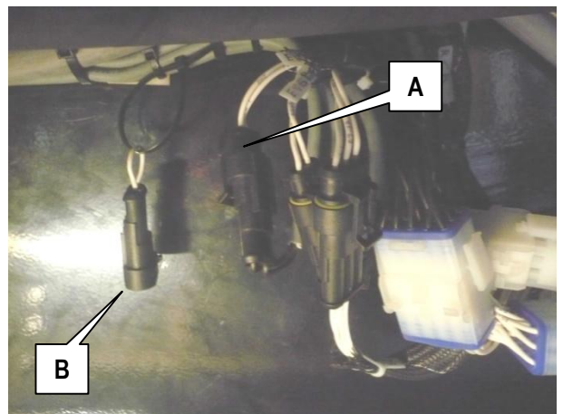
7-10: By-pass système de détection de surcharge
