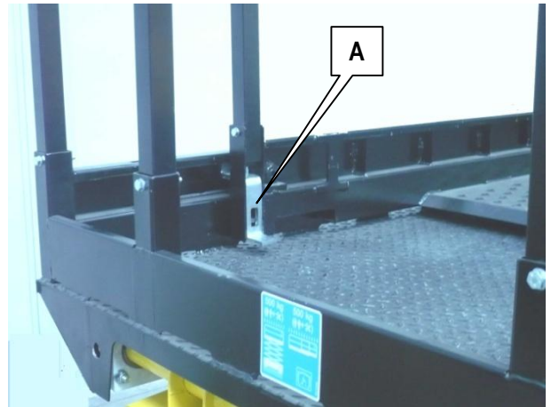
5-2: Pédale de déblocage extension plate-forme mobile
