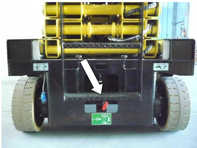
5-6: Descente manuelle d'urgence à un bouton
