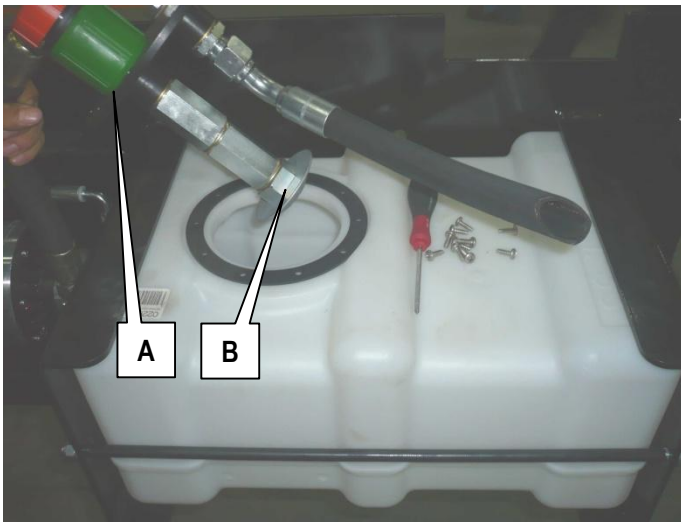
7-7: Réservoir série X
