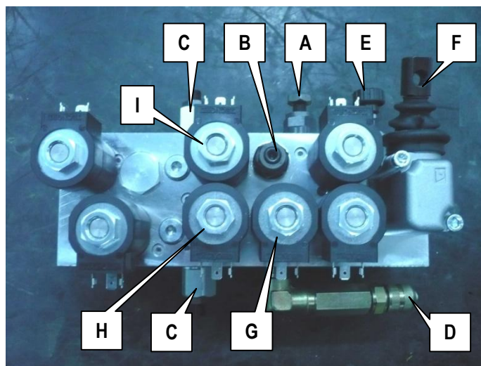
7-8: Bloc hydraulique
