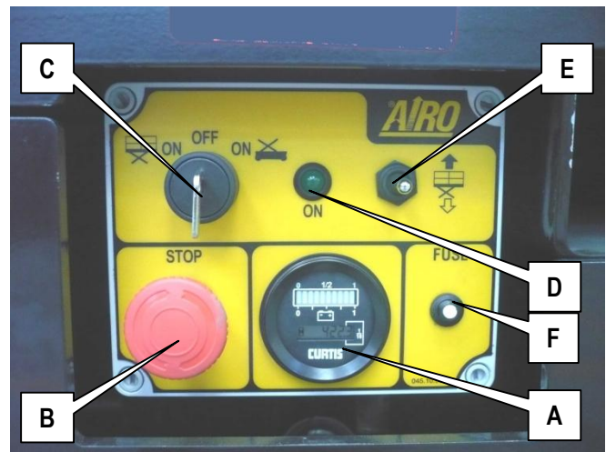
5-3: Tableau de commande au sol
