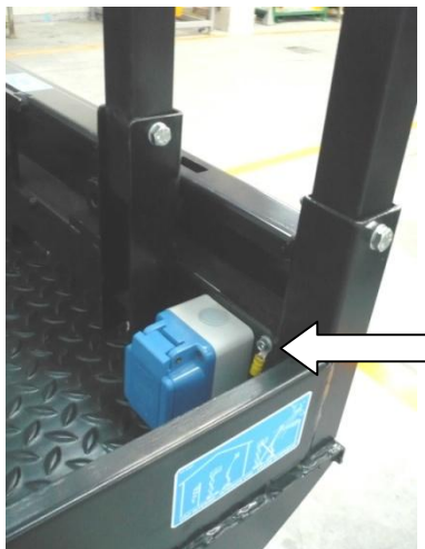
5-8: Prise de courant en haut
