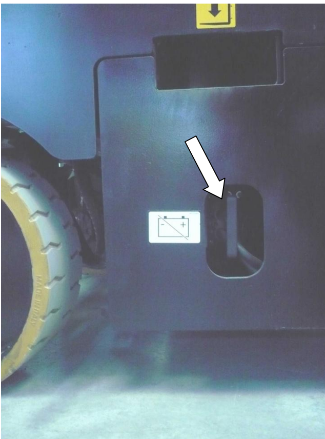
5-5: Connecteur de puissance série "X"
