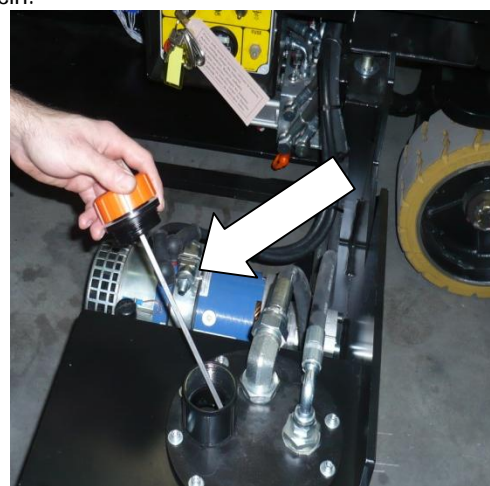
Bouchon de contrôle du niveau de l'huile de la série XSE RESTYLING
