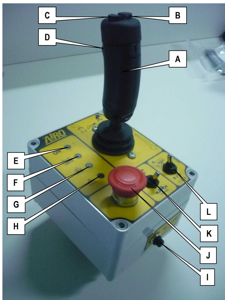
5-1: Tableau de commande de la plate-forme
