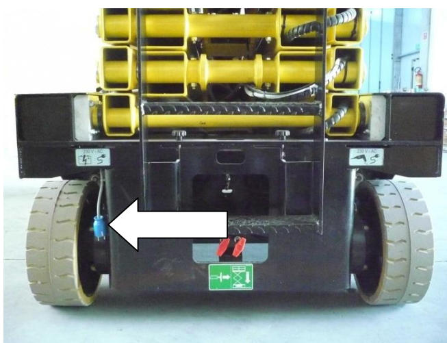
7-13: Fiche du chargeur de batterie
