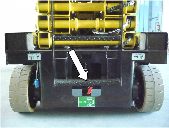
5-7: Descente manuelle d'urgence à un bouton
