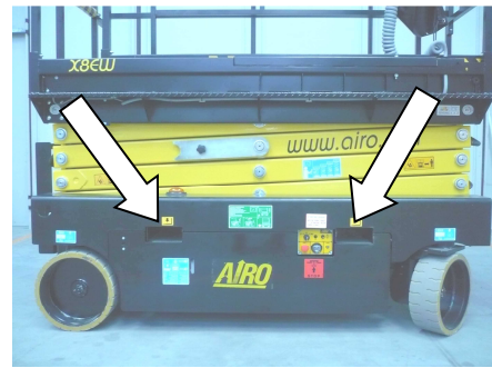
6-2: Cales pour fourches
