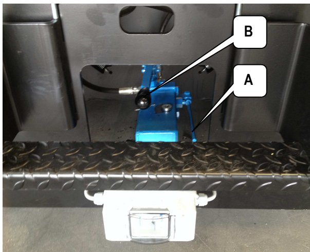
5-8: Descente manuelle du sol
