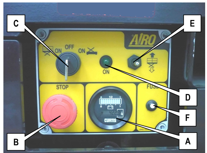
5-3: Tableau de commande au sol
