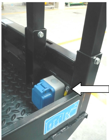
5-9: Prise de courant en haut
