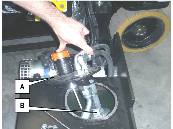
Réservoir série XS E RESTYLING
