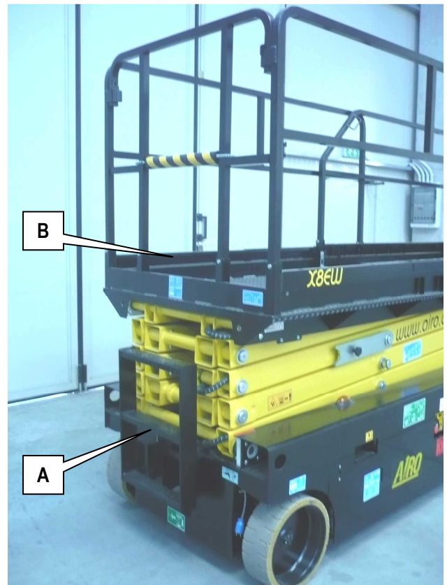
5-4: Position d'accès/abandon à la plate-forme
