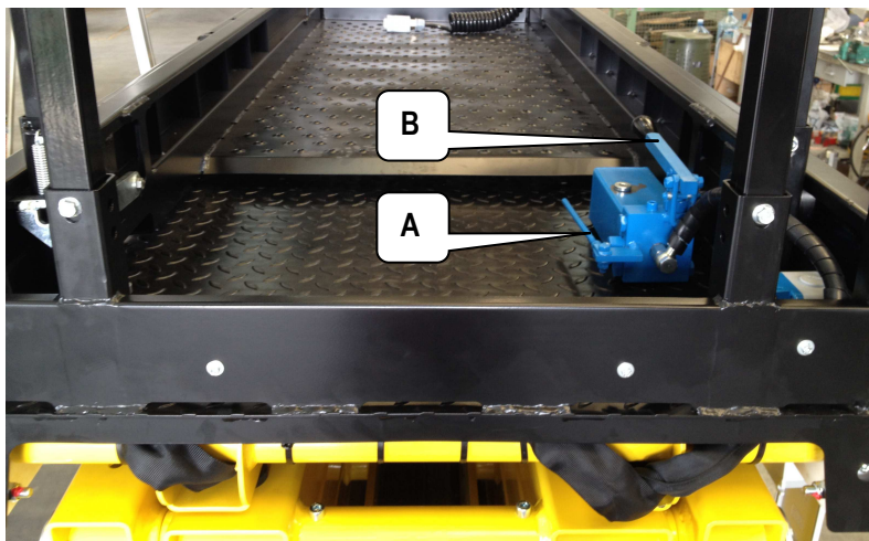
5-9: Descente manuelle de la plate-forme
