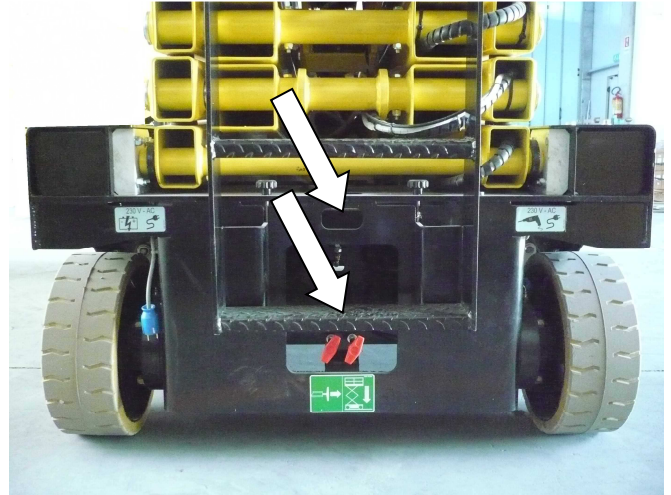
5-8: Descente manuelle d'urgence à deux boutons
