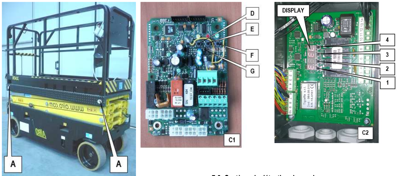
7-9: Système de détection de surcharge
