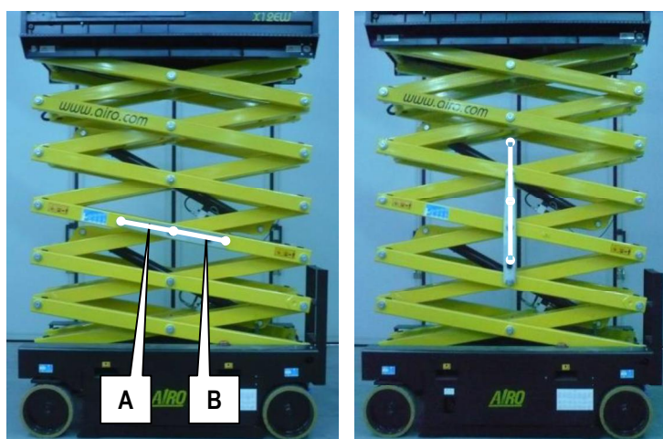
7-3: Bloccaggio forbice X12 EN, X12 EW, X12 EW-WIND, X14 EW, X99 E RESTYLING
