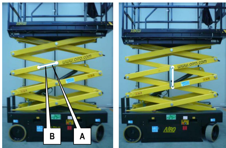
7-2: Bloccaggio forbice X10 EN, X10 EW, X10 EW-WIND, X88 E RESTYLING LIGHT, X88 E RESTYLING
