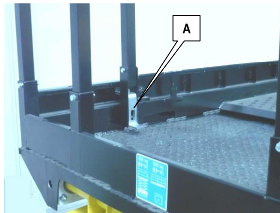
5-2: Pedale di sblocco sfilo piattaforma mobile
