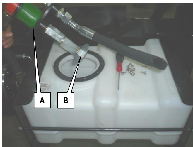
7-7: Serbatoio serie X
