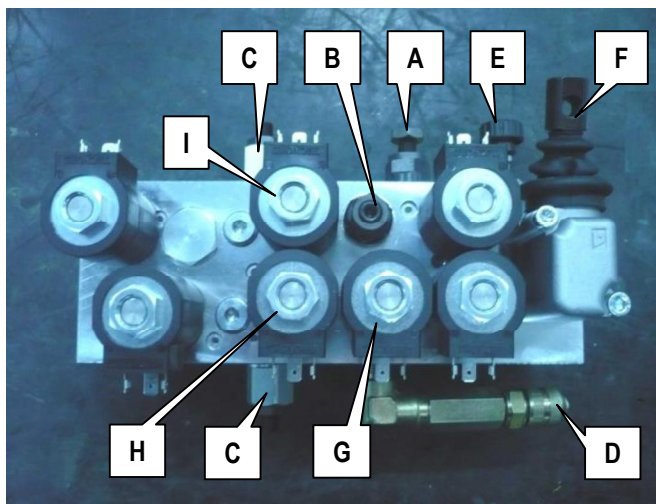
7-8: Blocco idraulico
