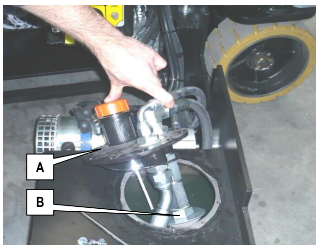
Serbatoio serie XS E RESTYLING
