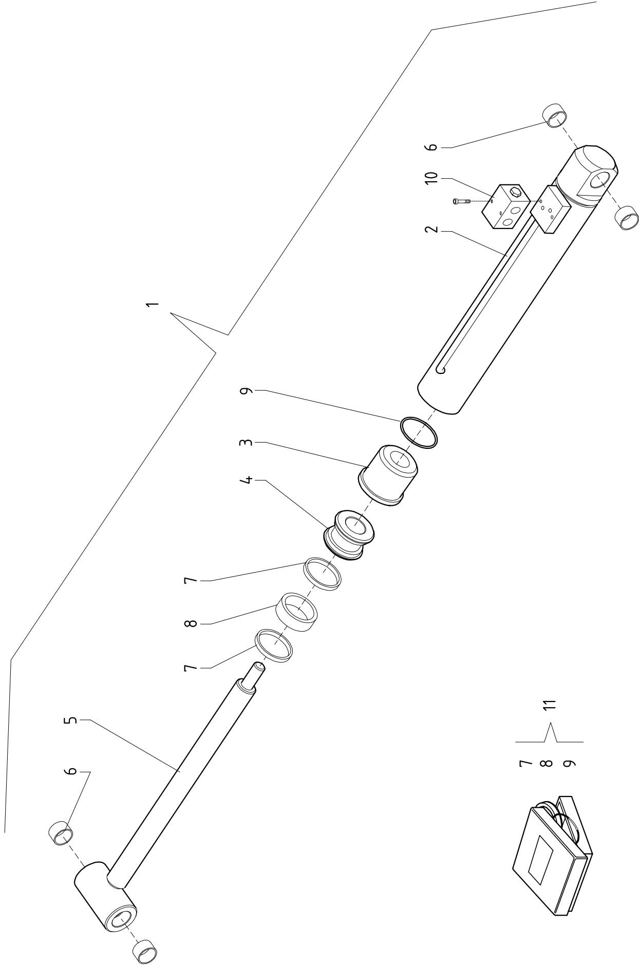
CILINDRO LIVELLAMENTO PIATTAFORMA (SLAVE) CAGE LEVELLING CYLINDER (SLAVE)
