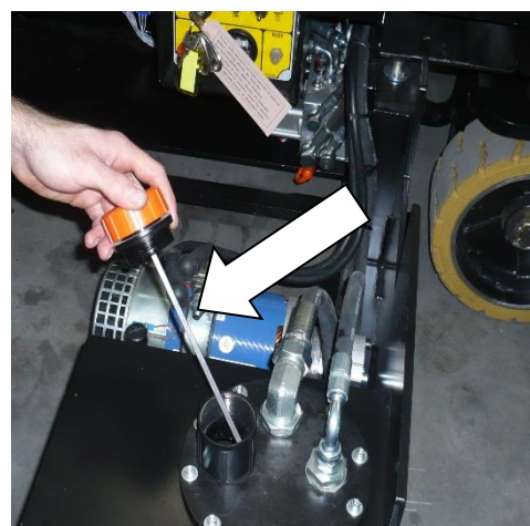
Dop de verificare a nivelului de ulei la seria XSE RESTYLING
