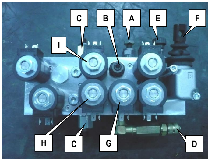
7-8: Bloc hidraulic
